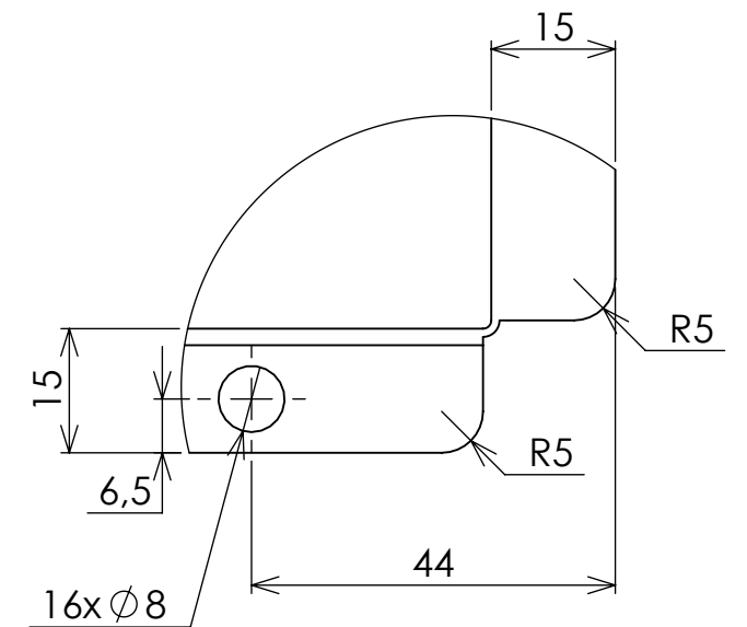
DETTAGLIO C
