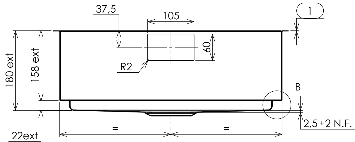
SEZIONE A-A
