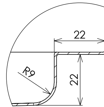
DETTAGLIO B
