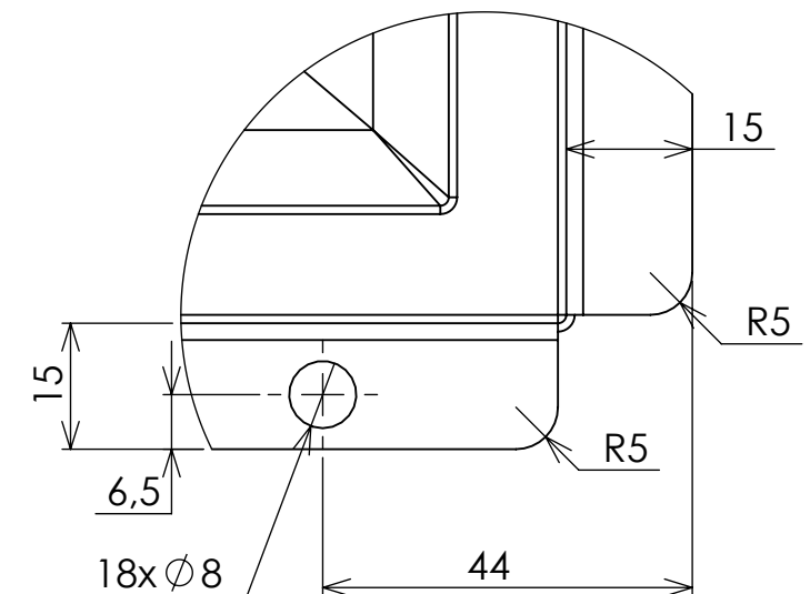
DETTAGLIO C
