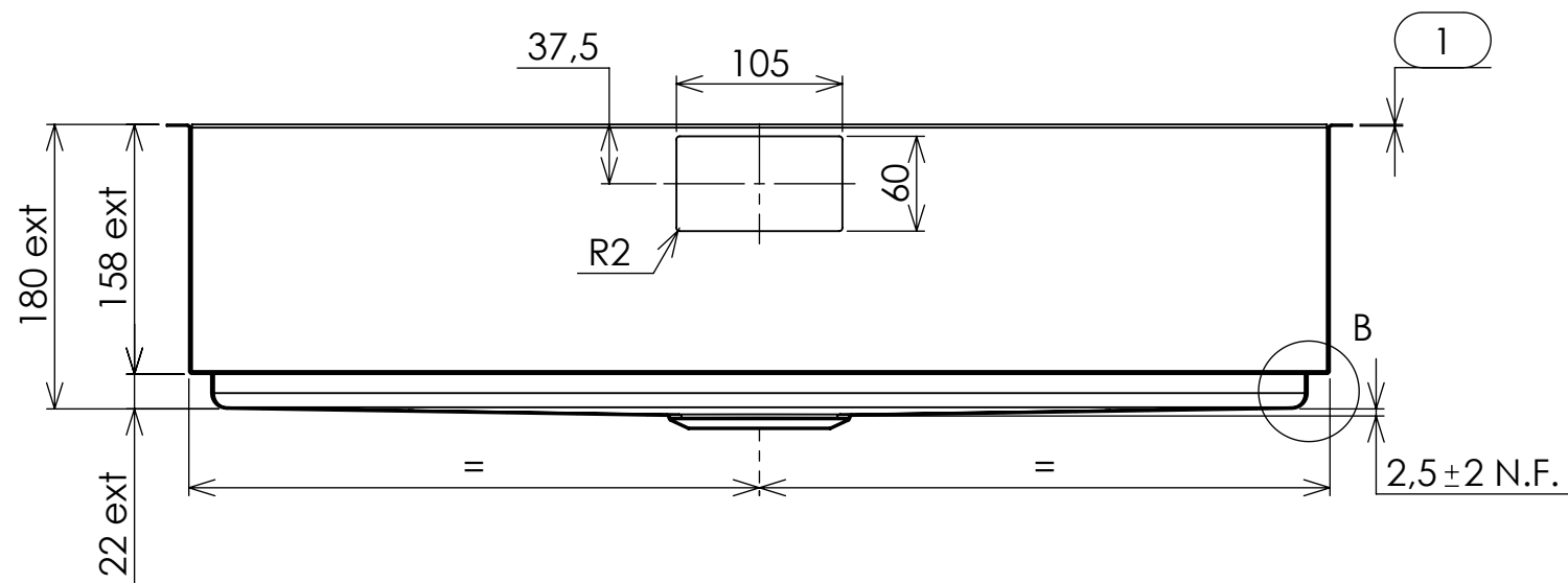
SEZIONE A-A
