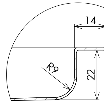
DETTAGLIO B
