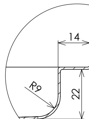
DETTAGLIO B
