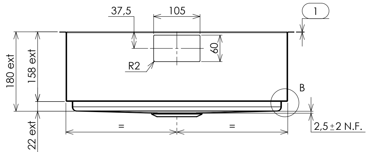
SEZIONE A-A
