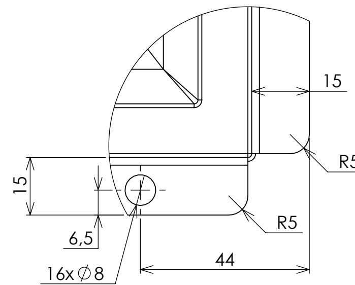
DETTAGLIO C
